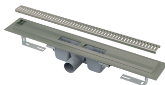
APZ1-N-B * Odpływ liniowy z perforowanym rusztem, NICKEL-mat szczotkowany
