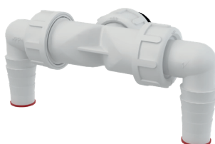
P155Z-G1 Podwójne kolano DN40/32 / 17-23 z zaworem
